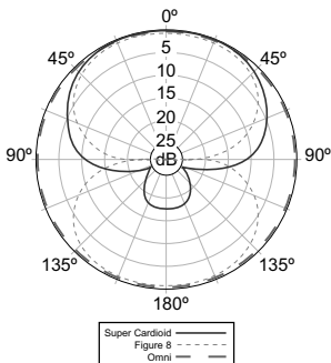
極特性線図
